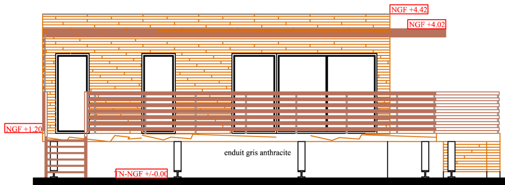
FACADE NORD
